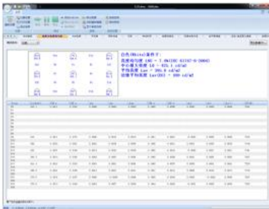
GAMMA 测试
